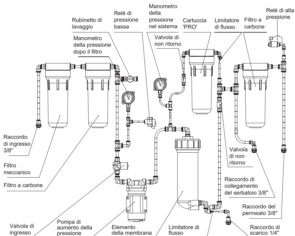
Figura 4. Schema del sistema Robust PRO (Codice: ROBUSTPROB)
